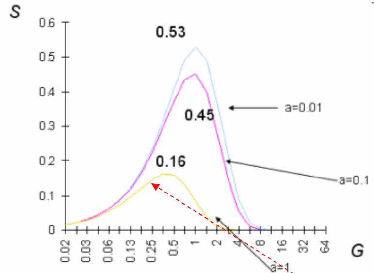
1-Persistent CSMA
